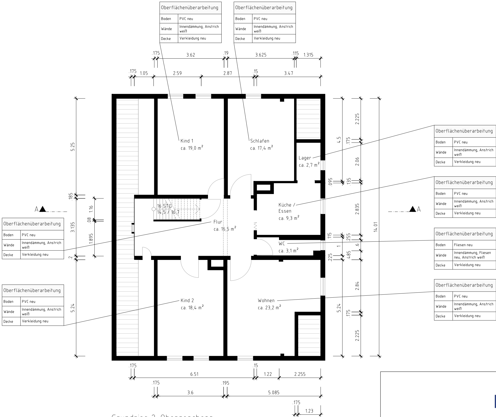
Grundriss 2. Obergeschoss
