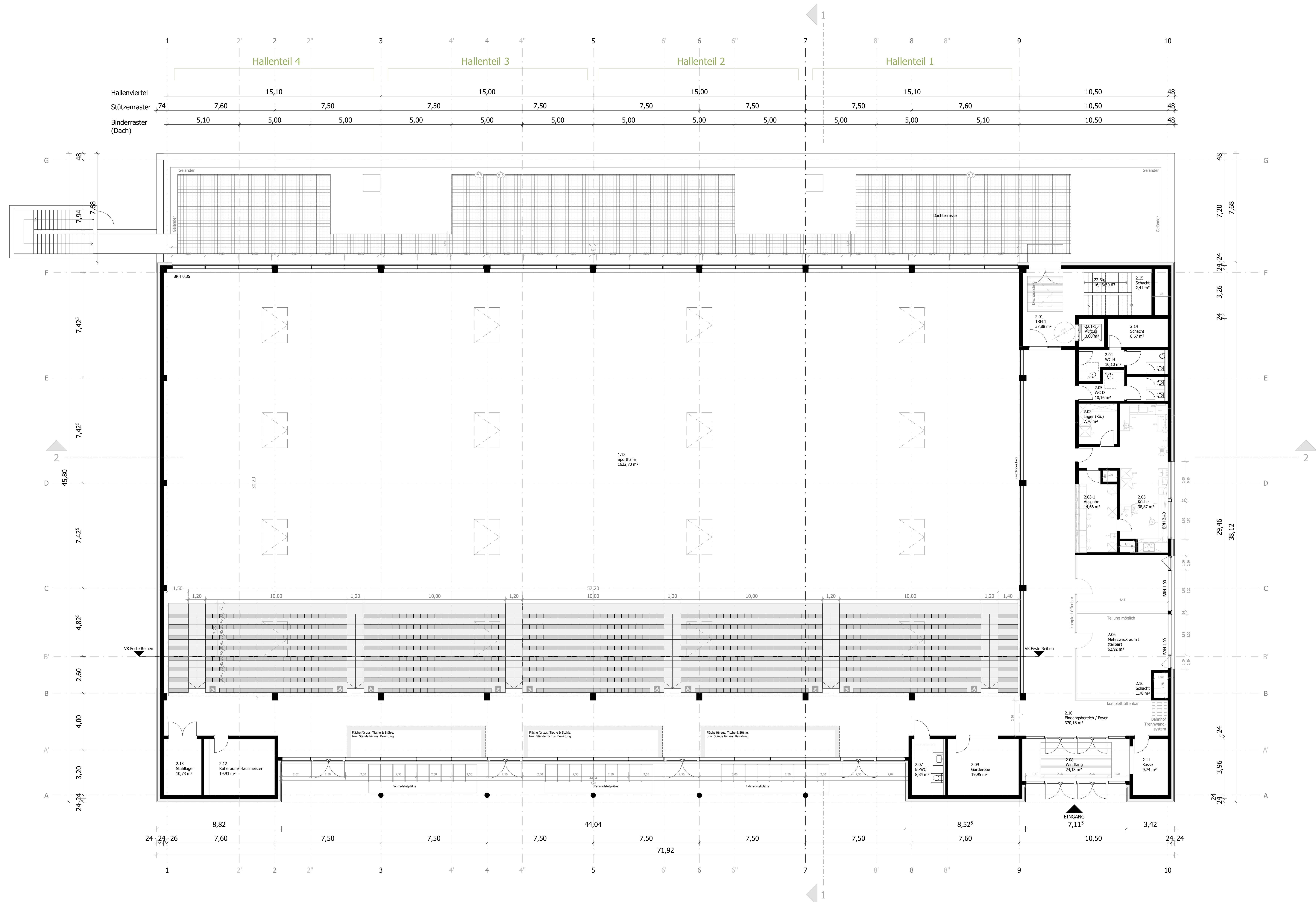
Grundriss Sporthalle, Ebene 00, Zuschauerebene mit Option Dachterrasse
