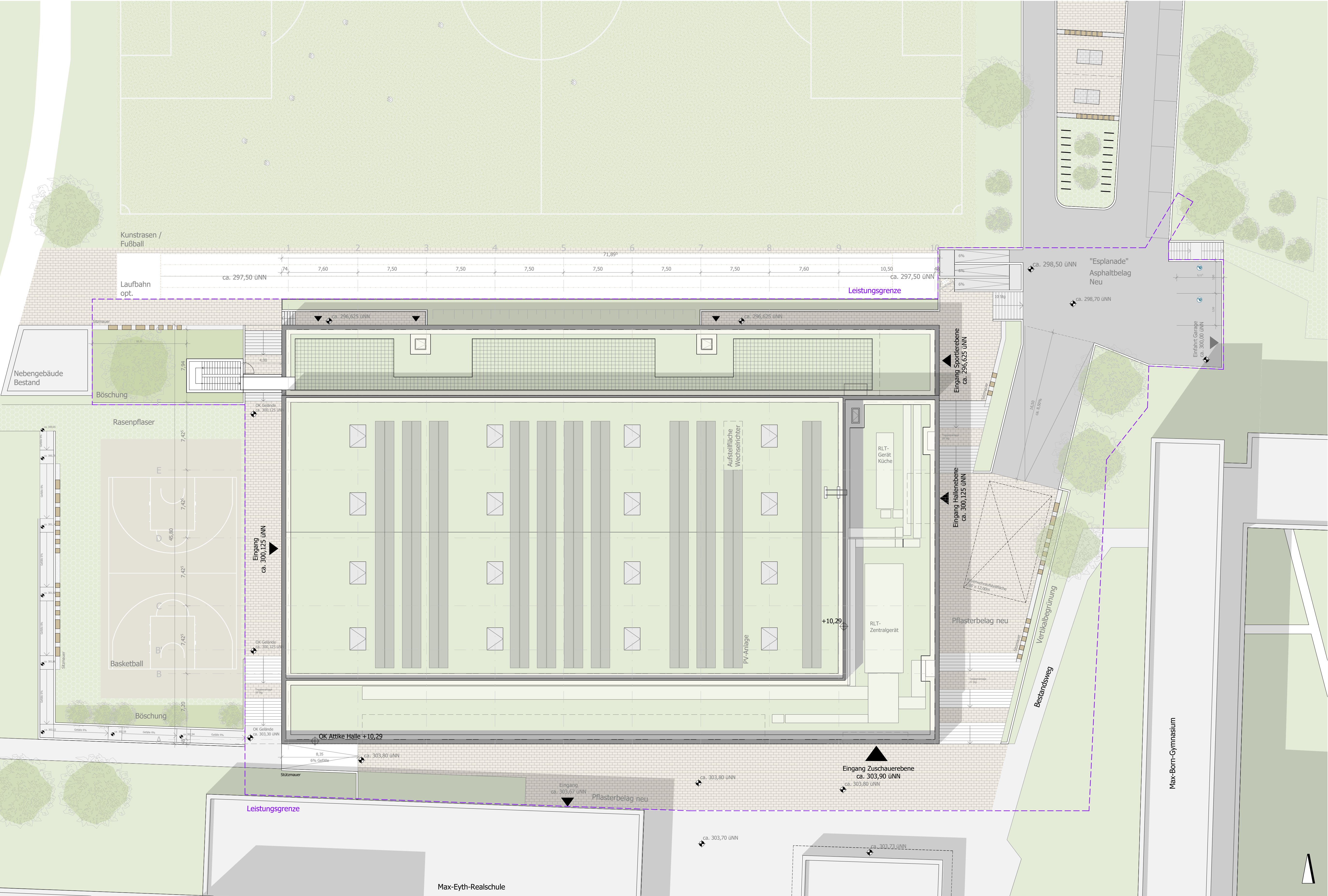
Lageplan Sporthalle, Außenanlagen - Dachaufsicht mit Option Dachterrasse
