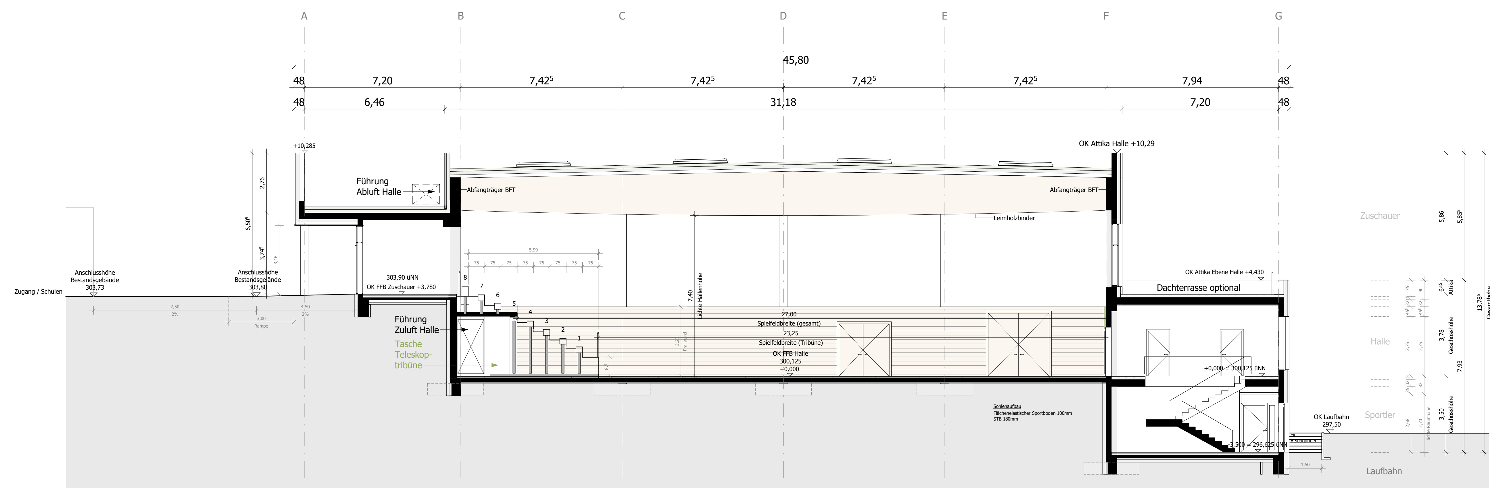
1-1 Querschnitt
