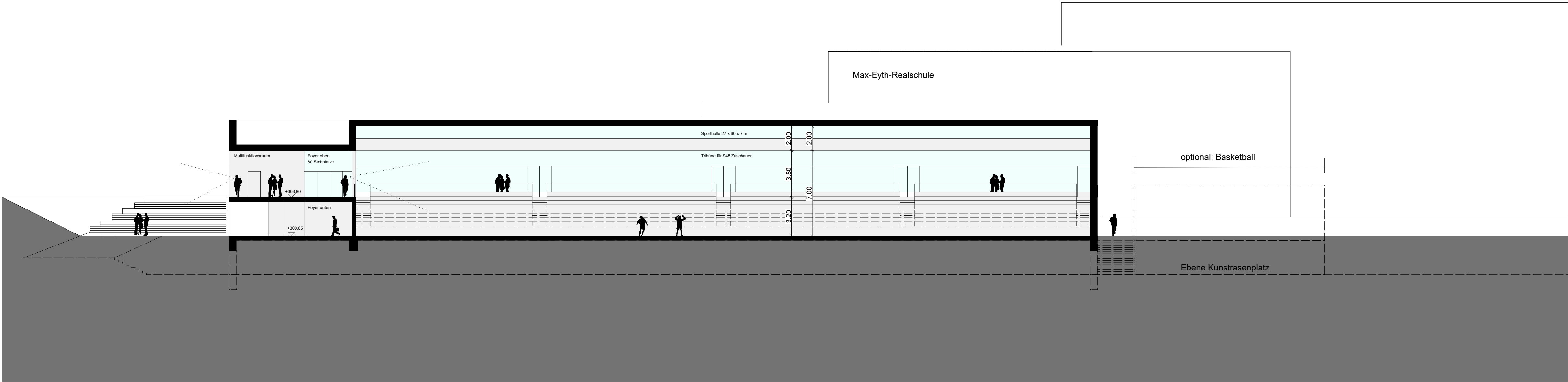
Längsschnitt Neubau
